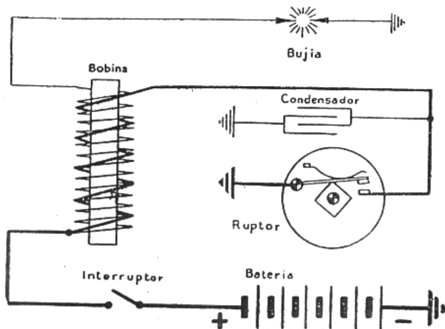
Esquema eléctrico de la instalación de encendido.
